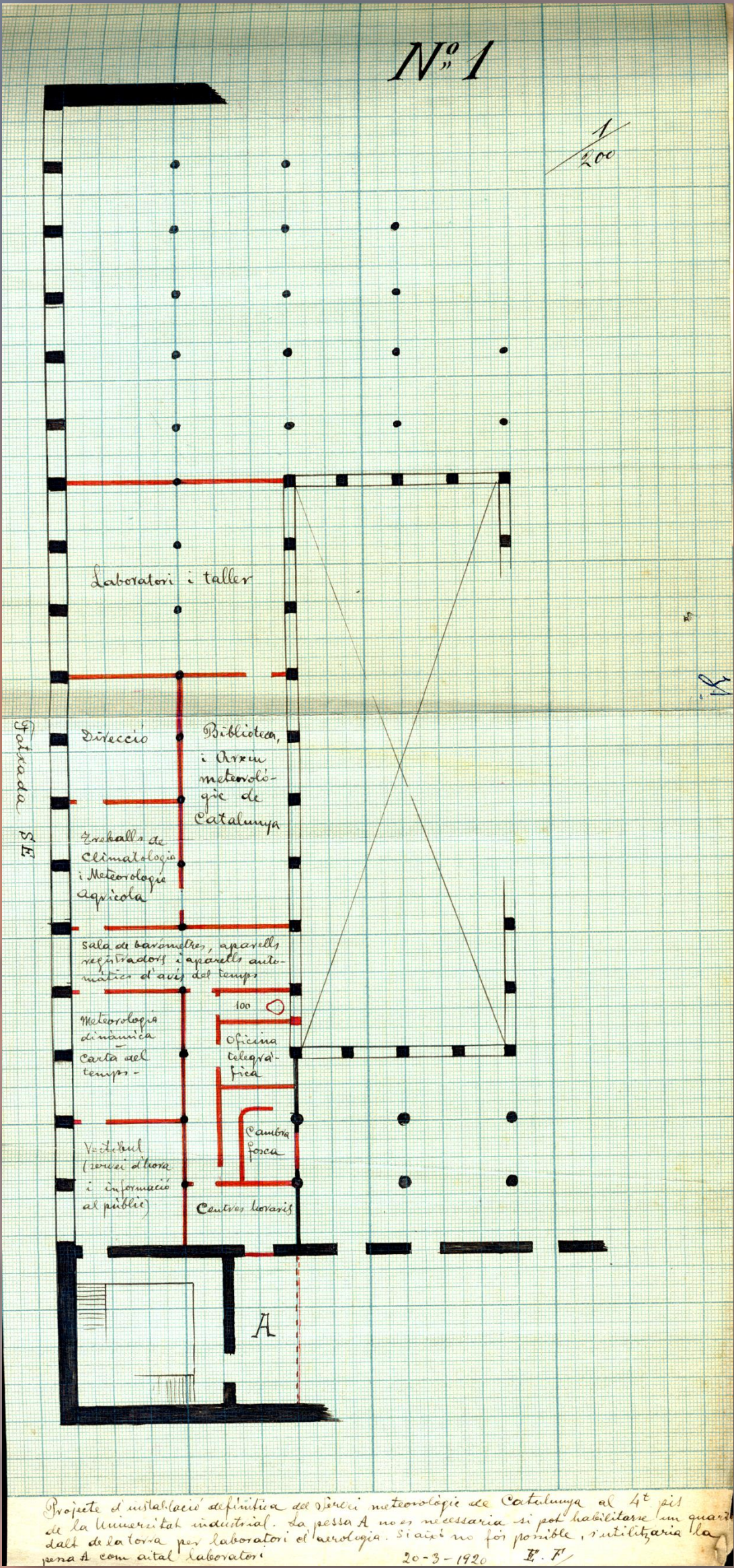
Plànol de distribució d'espais del primer Servei Meteorològic de Catalunya, al 4a planta de la Universitat Industrial.
